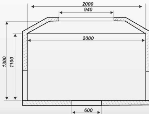
Przekrój podłużny
