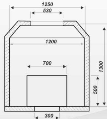
Przekrój poprzeczny
